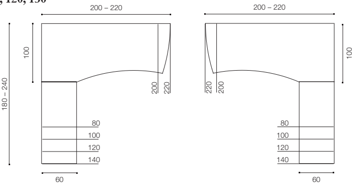
Tischkombination wahlweise Standardposition oder zurück gesetzt
