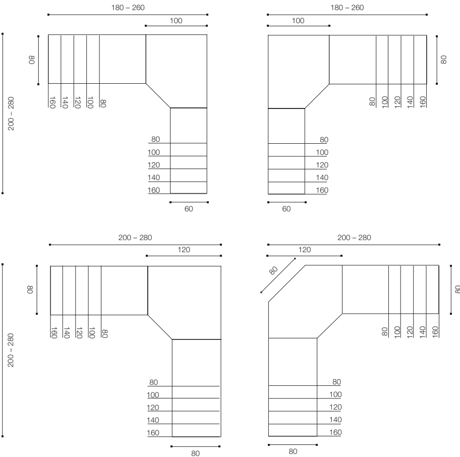
Tischkombination mit zurück gesetztem Fuß im Schwenkbereich
