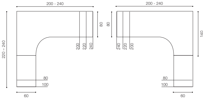
Tischkombination wahlweise Standardposition oder zurück gesetzt
