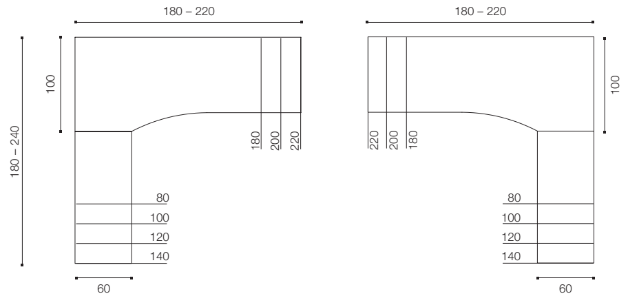
Tischkombination mit zurück gesetztem Fuß im Schwenkbereich
