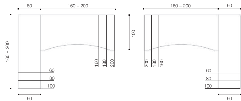
Tischkombination wahlweise Standardposition oder zurück gesetzt
