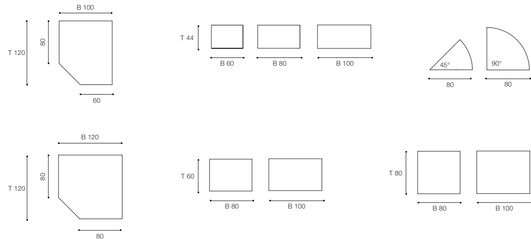
Verbindungselement nur in Verkettung mit Tisch, Anstellkorpus oder Schrank. Verkabelung wahlweise mit Metalkabelkanal
