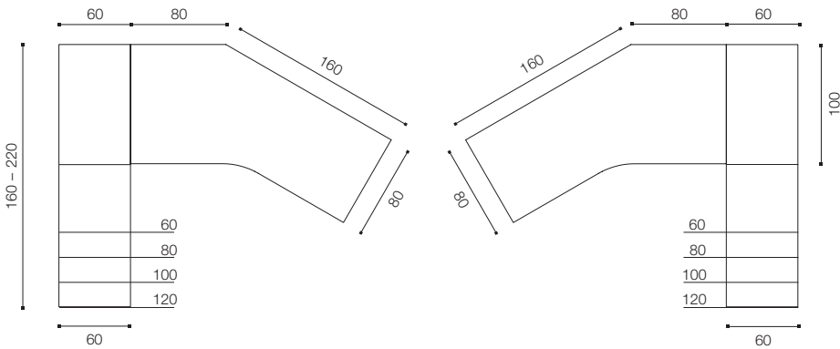
Tischkombination wahlweise Standardposition oder zurück gesetzt
